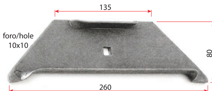
Angolare per reti Frame corner Cod.: ANB26580
